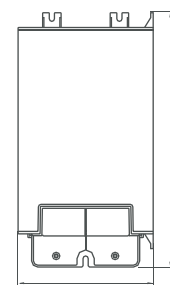
LxWxH : 207x110x44.8mm
